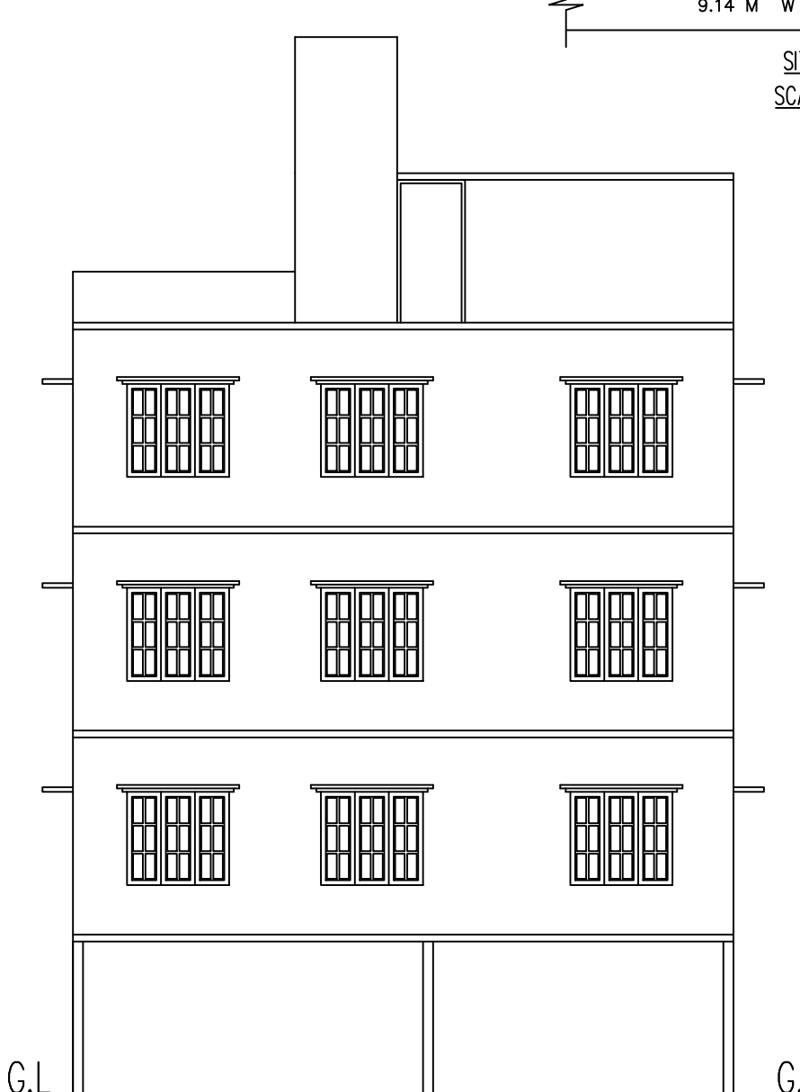
ELEVATION
